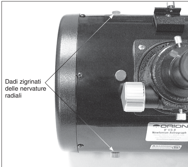
Figura 12. Per centrare lo specchio secondario lungo il raggio nel tubo interno del focheggiatore, regolare le due viti zigrinate delle nervature radiali perpendicolari al focheggiatore.
