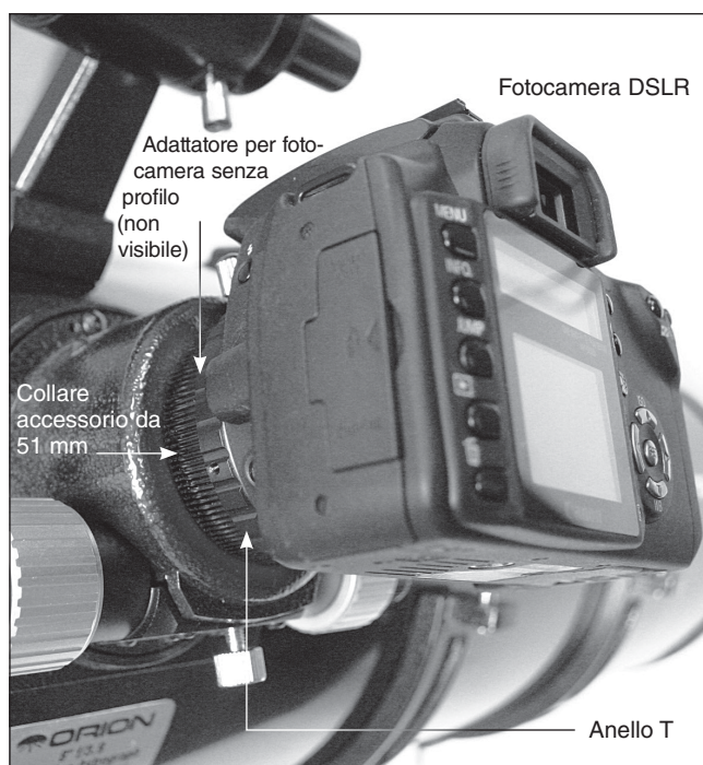
Figura 6. Il fissaggio di una fotocamera DSLR richiede un anello T per il particolare modello di fotocamera e un adattatore a T, come l'adattatore per fotocamera con fuoco primario senza profilo di Orion, da inserire nel collare accessorio da 51 mm.
