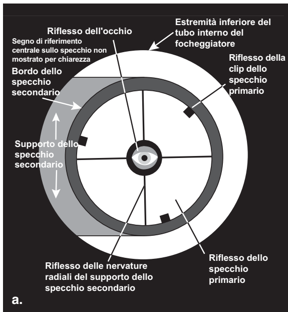
Figura 8. Collimazione delle ottiche. (a) Se gli specchi sono allineati correttamente, l'immagine attraverso il tubo interno del focheggiatore dovrebbe assomigliare a quella illustrata. (b) Con il tappo di collimazione applicato, se l'ottica non è allineata, l'immagine potrebbe assomigliare a quella illustrata. (c) In questo caso lo specchio secondario è centrato sotto il focheggiatore, ma deve essere regolato (inclinato) in modo che l'intero specchio primario sia visibile. (d) Lo specchio secondario è allineato correttamente, ma lo specchio primario ha ancora bisogno di regolazione. Quando lo specchio primario è allineato correttamente, il punto centrale del tappo di collimazione risulta centrato, come in (e) .
