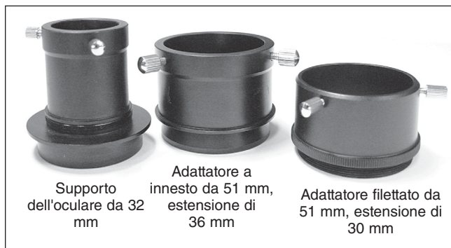
Figura 7. Il supporto dell'oculare da 32 mm e i due adattatori di estensione da 51 mm inclusi con gli astrografi Newton da 203 mm e 254 mm e rapporto focale f/3,9.
