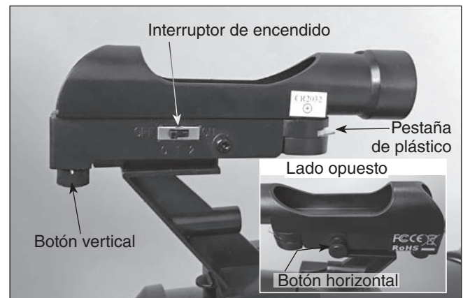
Figura 12. El telescopio buscador de punto rojo tiene botones de ajuste vertical y horizontal (insertado) para alinearlos con el telescopio.
