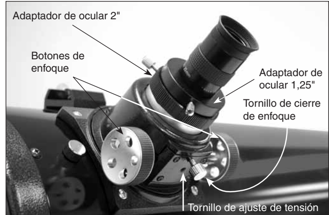
Figura 10. El enfocador Crayford de 2" (XT8 y XT10)
